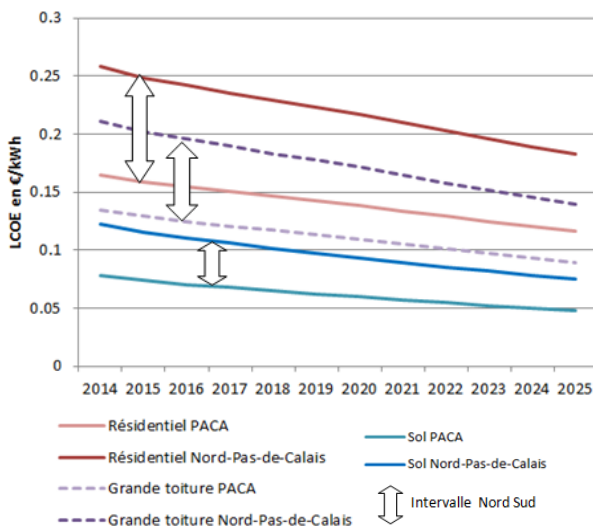
Evolution du coût de production du kWh photovoltaïque (LCOE)
